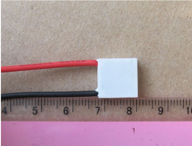
Figure 1.1. The Photo of Actual ATE1-17
