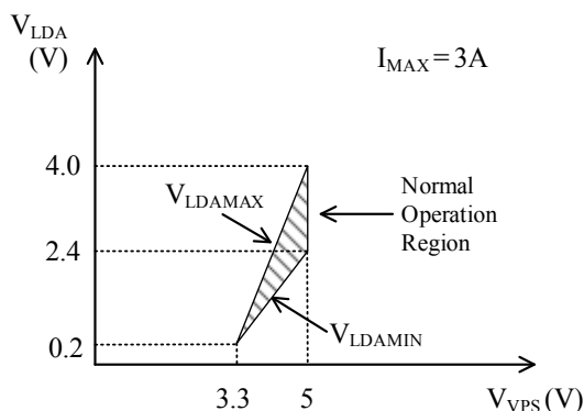
Figure 6. V_{VPS} & V_{LDA}
